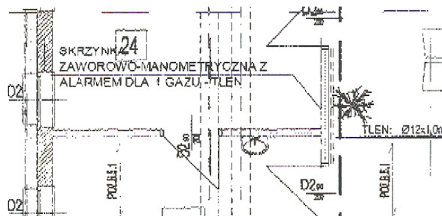
wycinek z rzutu II piętra rysunku instalacji gazów medycznych nr GM-04
